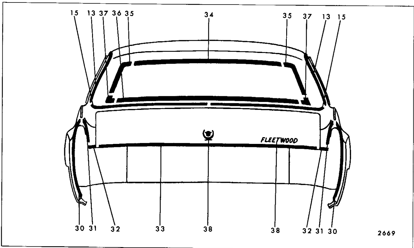
Fig. 17-121—Cadillac 68069-68169 Styles
